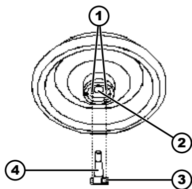
Abb. 16: Ein-Ausbau Rotor
