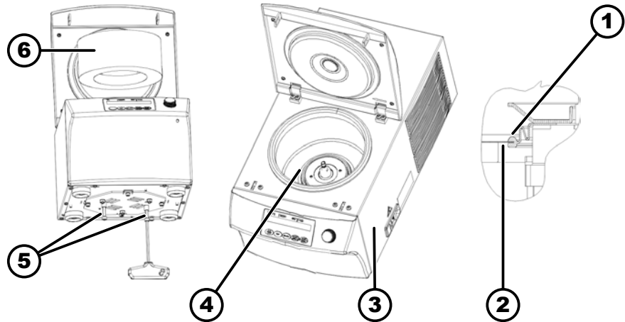
Abb. 13: Transportsicherung
