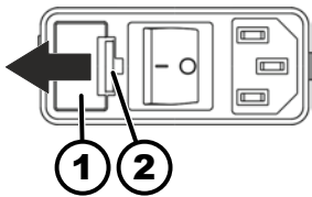
Abb. 19: Netzeingangssicherung
