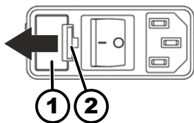
Fig. 19 : Fusible d'entrée du réseau
