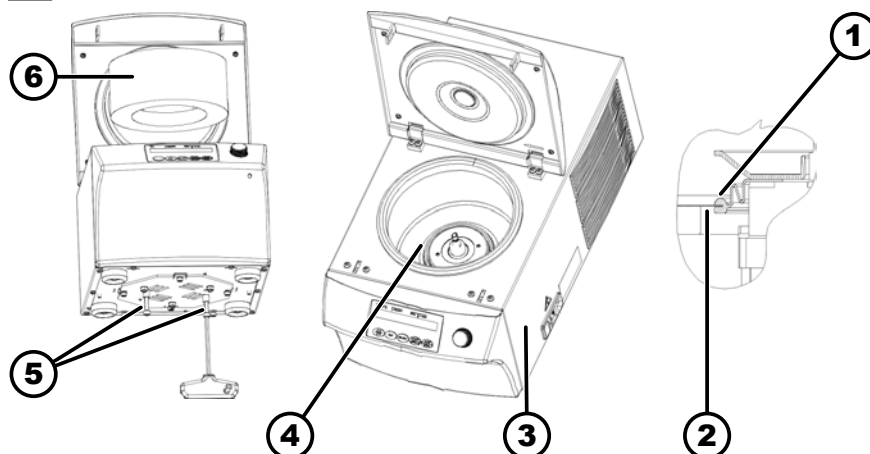
Abb. 14: Transportsicherung
