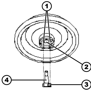
Kuva 16: Roottorin asennus ja irrotus
