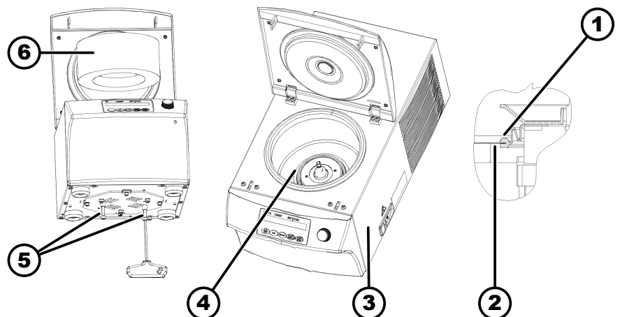
Kuva 13: Kuljetusvarmistin
