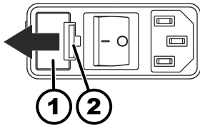
Kuva 19: Verkon tulovaroke
