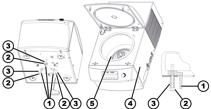
插图 14: 运输固定装置
