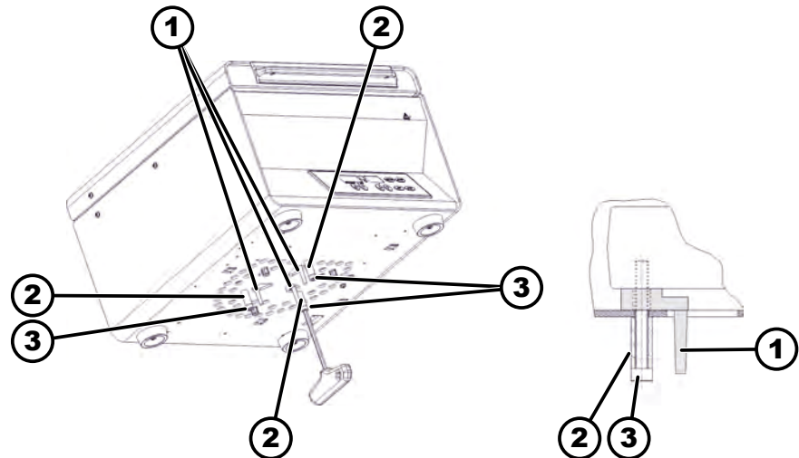
Abb. 14: Transportsicherung
