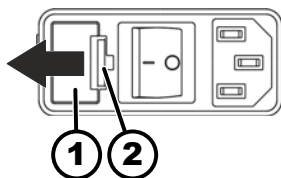
Abb. 21: Netzeingangssicherung
