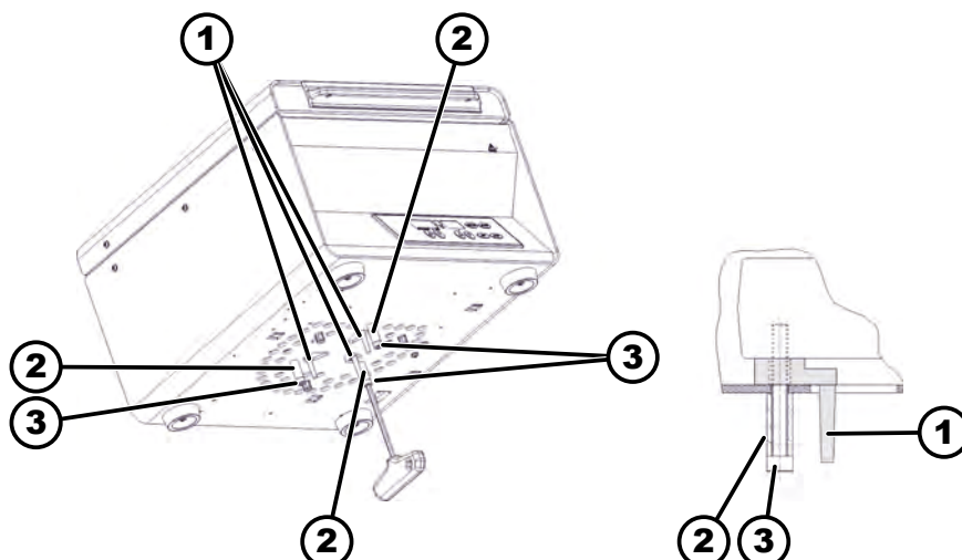
Abb. 13: Transportsicherung
