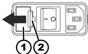
Απεικ. 21: Ασφάλεια εισόδου τροφοδοσίας
