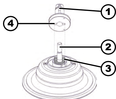
Απεικ. 17: Τοποθέτηση και αφαίρεση πλήμνης
