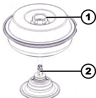
Fig. 16: Montar e desmontar o rotor
