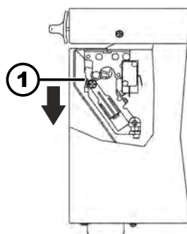
Απεικ. 20: Απασφάλιση έκτακτης ανάγκης
