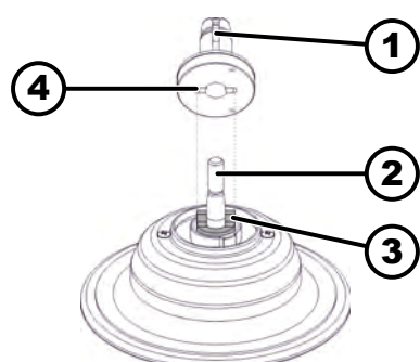
Fig. 17: Montar e desmontar o cubo
